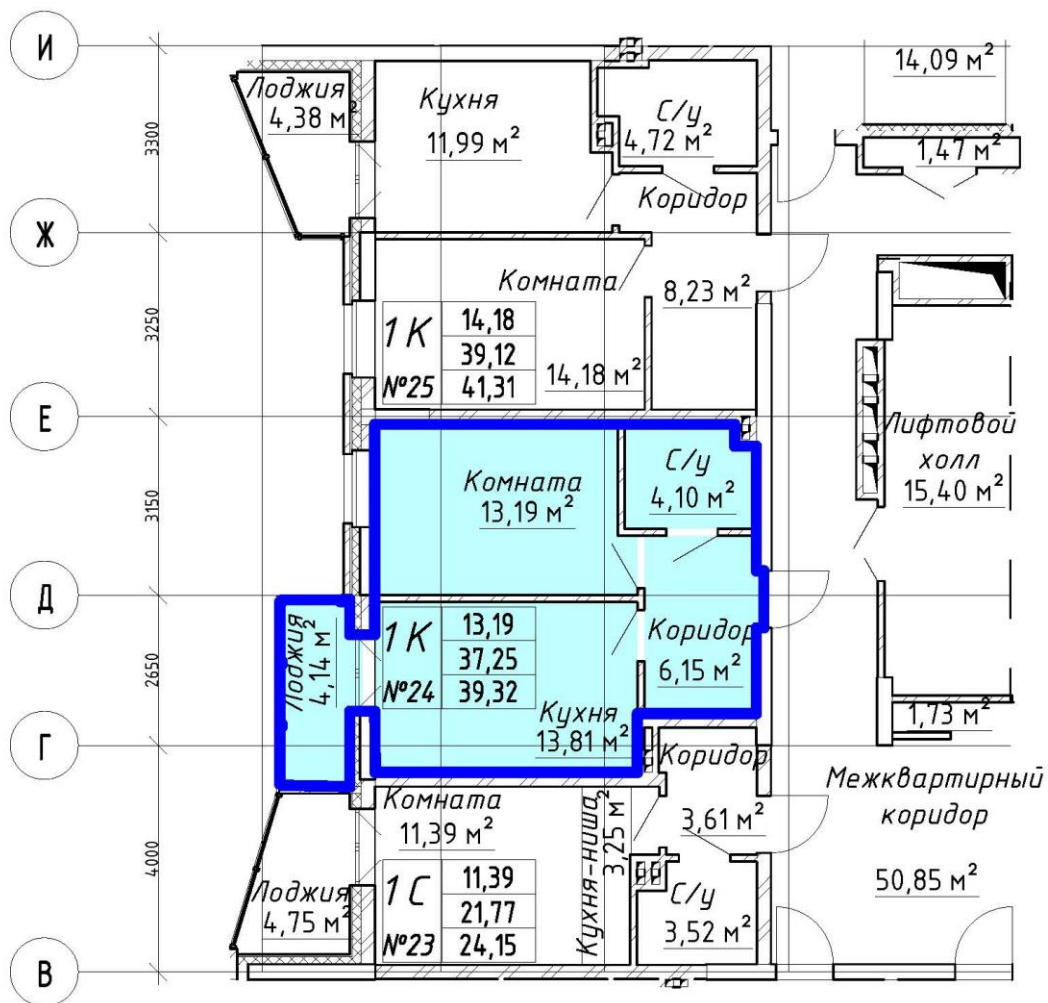
Экспликация к поэтажному плану здания (строения)
